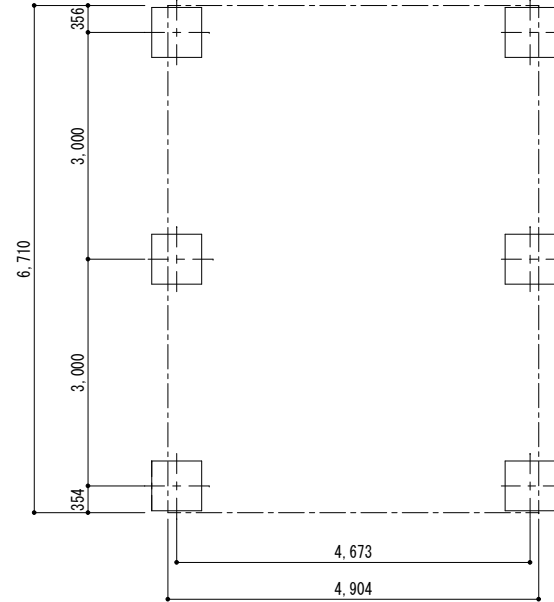
■基礎配置図
